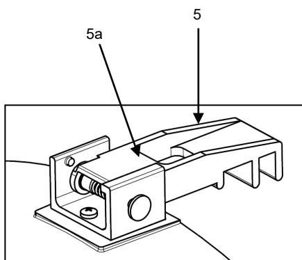
Klappbare Torsicherung / top latch
