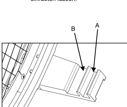
Halteklauen / accessory brackets
